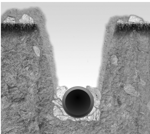
Фрагмент укладки трубы с защитным слоем в каменистом грунте
